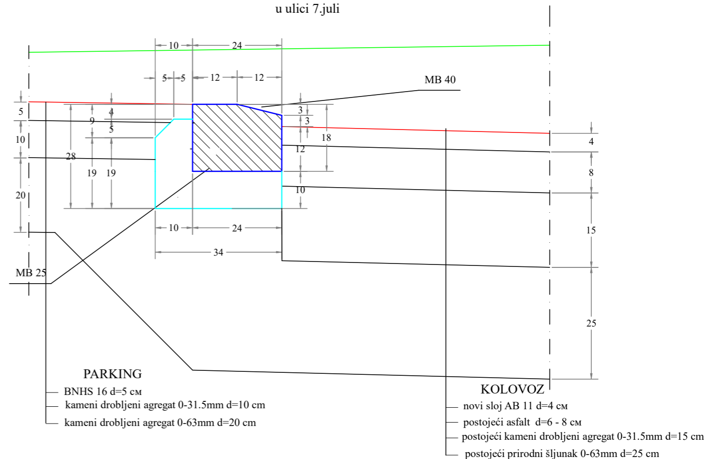
DETALJ POSTAVLJANJA IVIČNJAKA 12/18 u ulici 7.juli iza parkinga i trotoara
