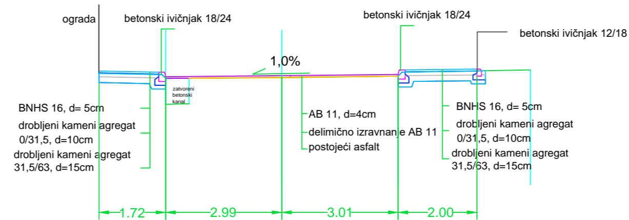
Карактеристични попречни профил 25 до 35
