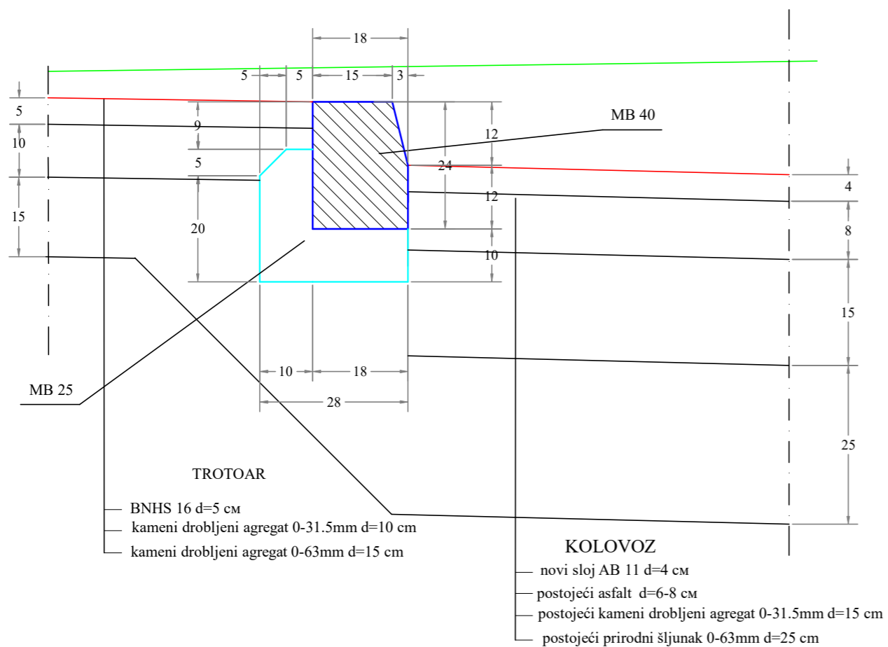
DETALJ POSTAVLJANJA IVIČNJAKA 18/24 u ulici 7.juli
