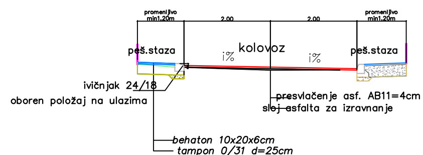
NORMALAN PROFIL Ivana Milutinovića km 0+630- km 0+662,35
