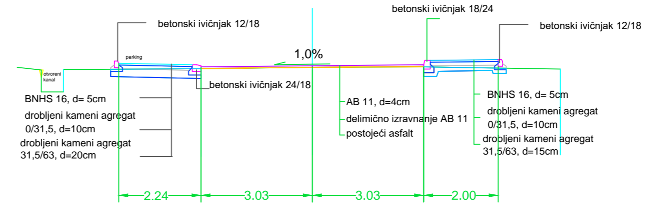
Карактеристични попречни профил 15 до 25
