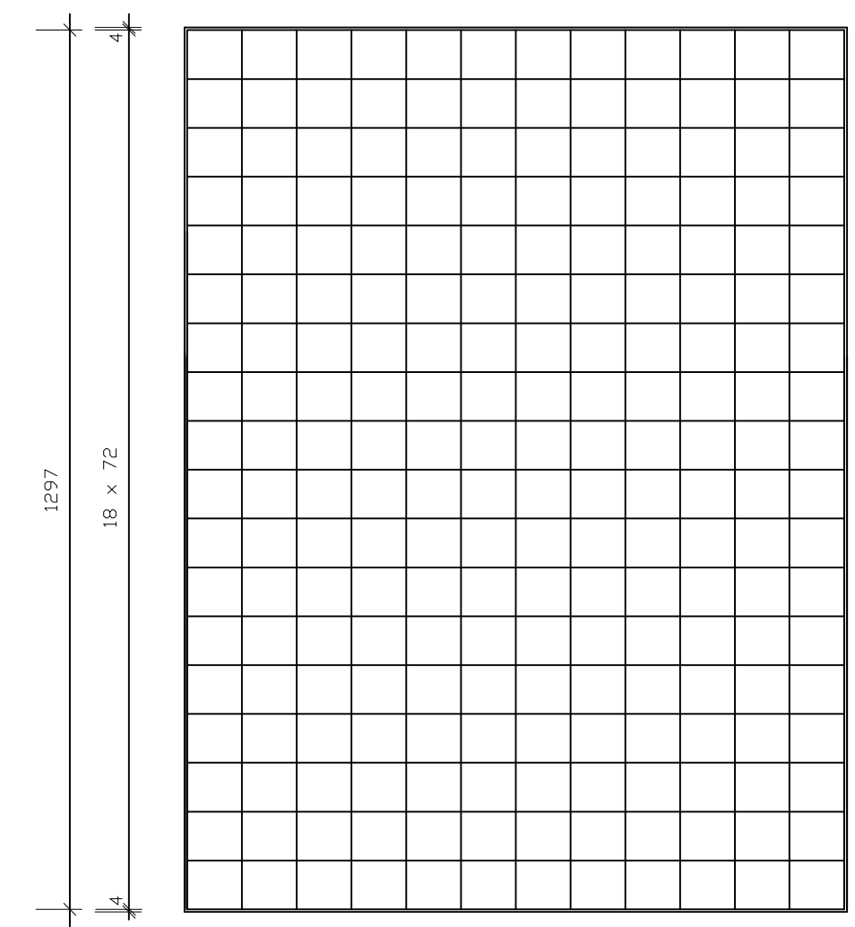
ДЕТАЉ РЕШЕТКЕ 97.00 x 129.70
