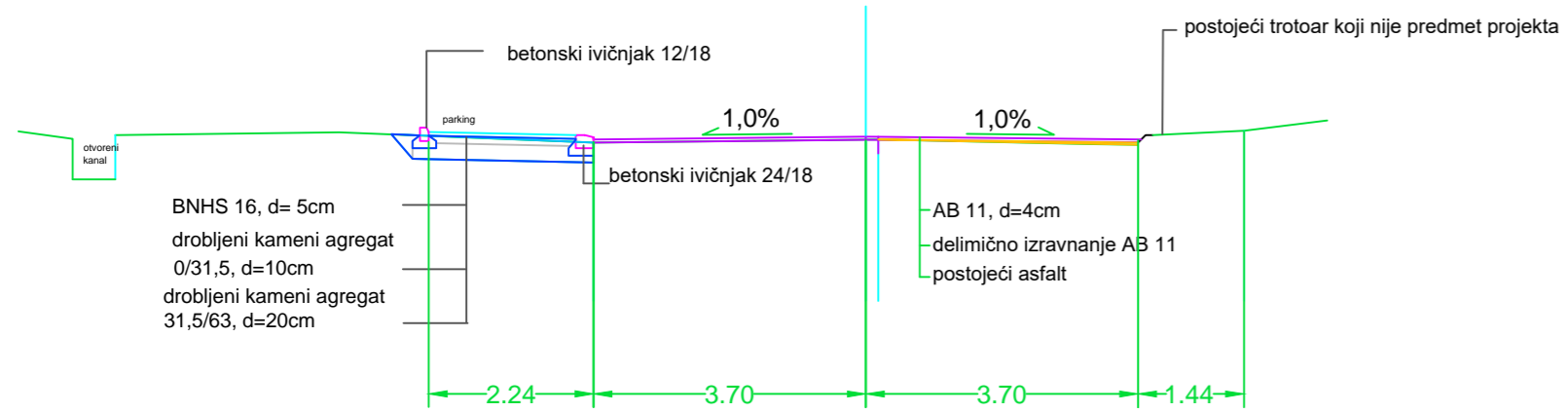
Карактеристични попречни профил 1 до 5
