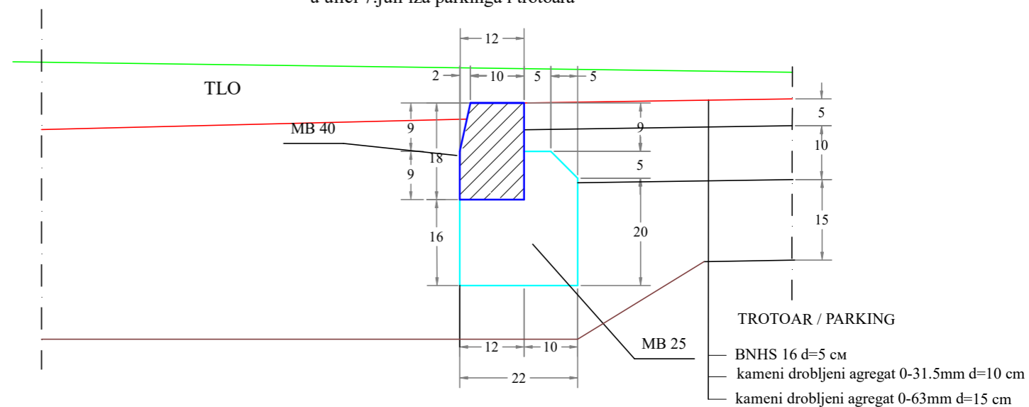
DETALJ POSTAVLJANJA IVIČNJAKA 12/18 u ulici 7.juli iza parkinga i trotoara
