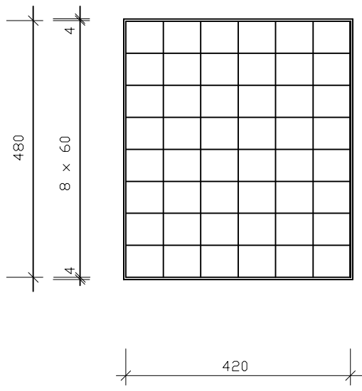
ДЕТАЉ РЕШЕТКЕ 42.00 x 48.00
