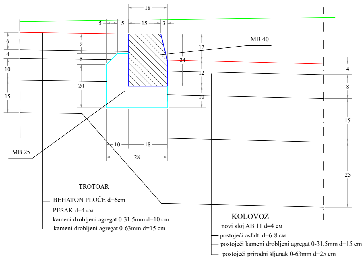
DETALJ POSTAVLJANJA IVIČNJAKA 18/24 u ulici 7.juli
