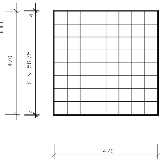
ДЕТАЉ РЕШЕТКЕ 47.00 x 47.00
