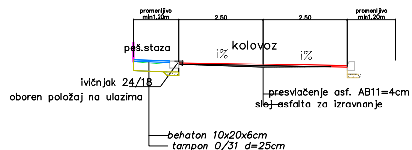
NORMALAN PROFIL Ivana Milutinovića km 0+214.46- km 0+630
