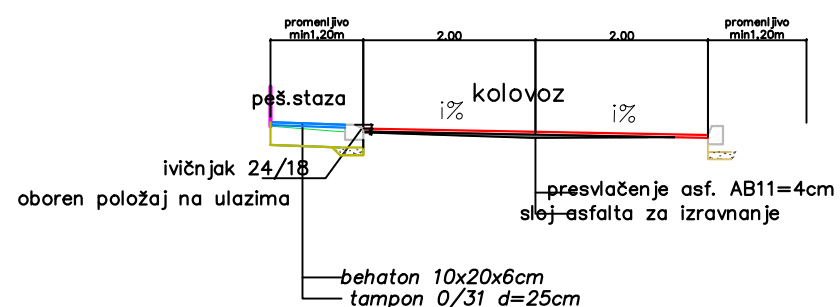
NORMALAN PROFIL Ivana Milutinovića km 0+003.00- km 0+074.00
