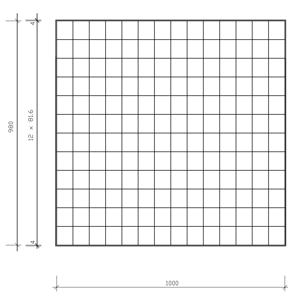
ДЕТАЉ РЕШЕТКЕ 100.00 x 98.00
