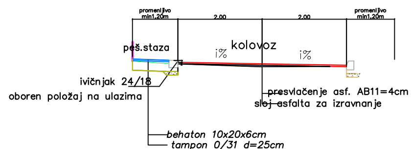
NORMALAN PROFIL Ivana Milutinovića km 0+074.00- km 0+214.46
