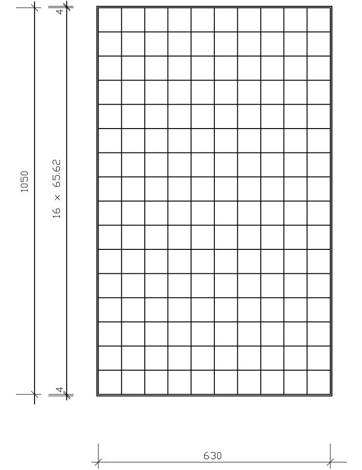
ДЕТАЉ РЕШЕТКЕ 63.00 x 105.00
