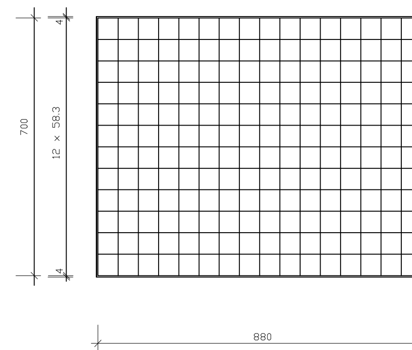
ДЕТАЉ РЕШЕТКЕ 88.00 x 70.00
